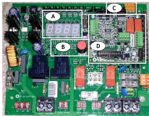
Rysunek 5.1 Płyta elektroniczna zainstalowana w GAHP (S61+Mod10)
