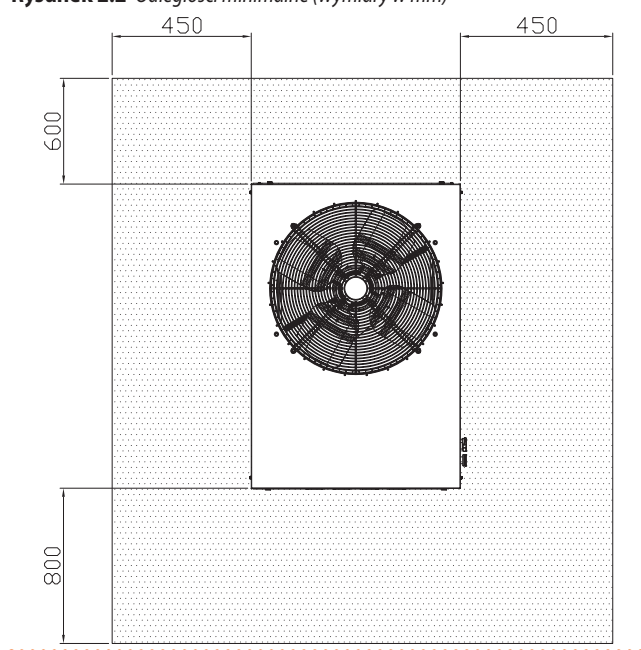
Rysunek 2.2 Odległości minimalne (wymiary w mm)
