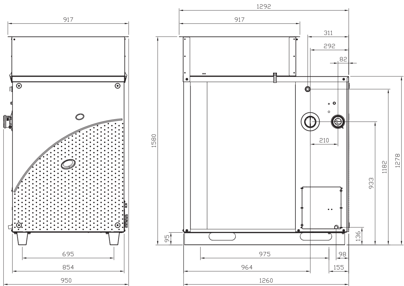
Rysunek 1.2 Wymiary GAHP-A indoor
