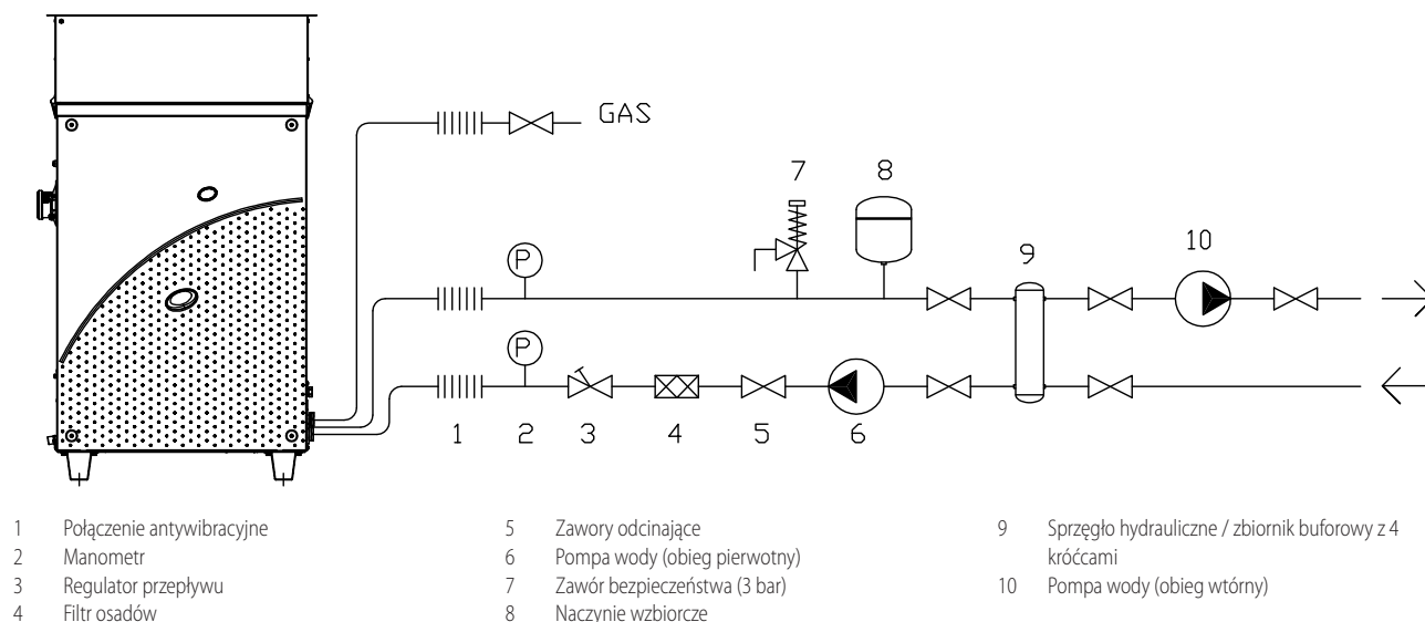
Rysunek 3.1 Schemat hydrauliczny
