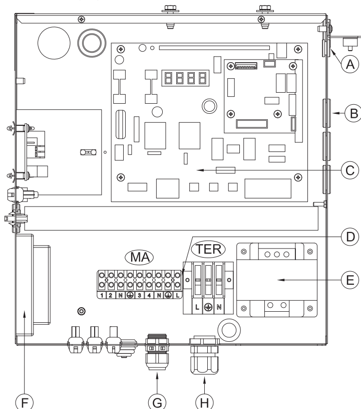
Rysunek 4.1 Panel elektryczny
