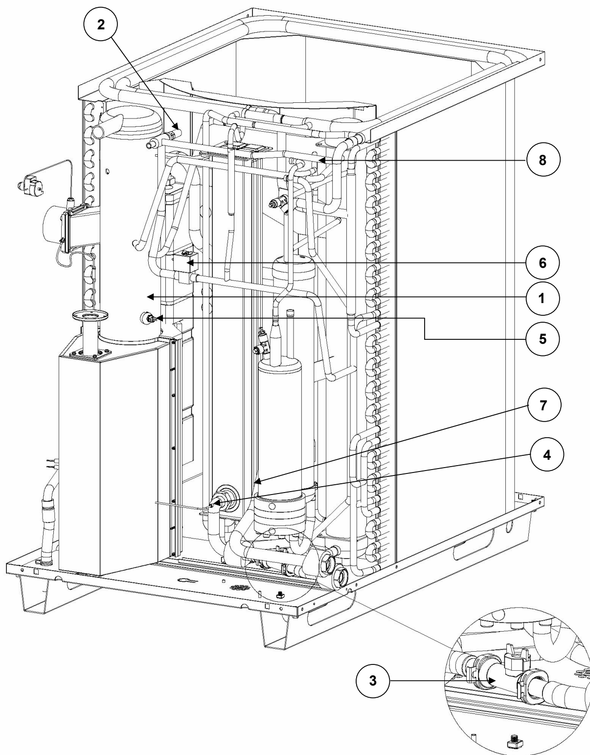
Rysunek 1.5 Elementy wewnętrzne - widok z prawej
