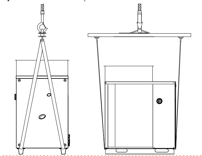
Rysunek 2.1 Podnoszenie urządzenia
