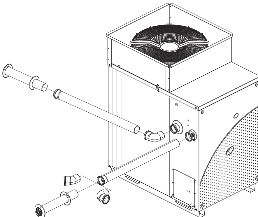
Rysunek 3.2 Odprowadzenie spalin Typu C53, układ rozdzielny
