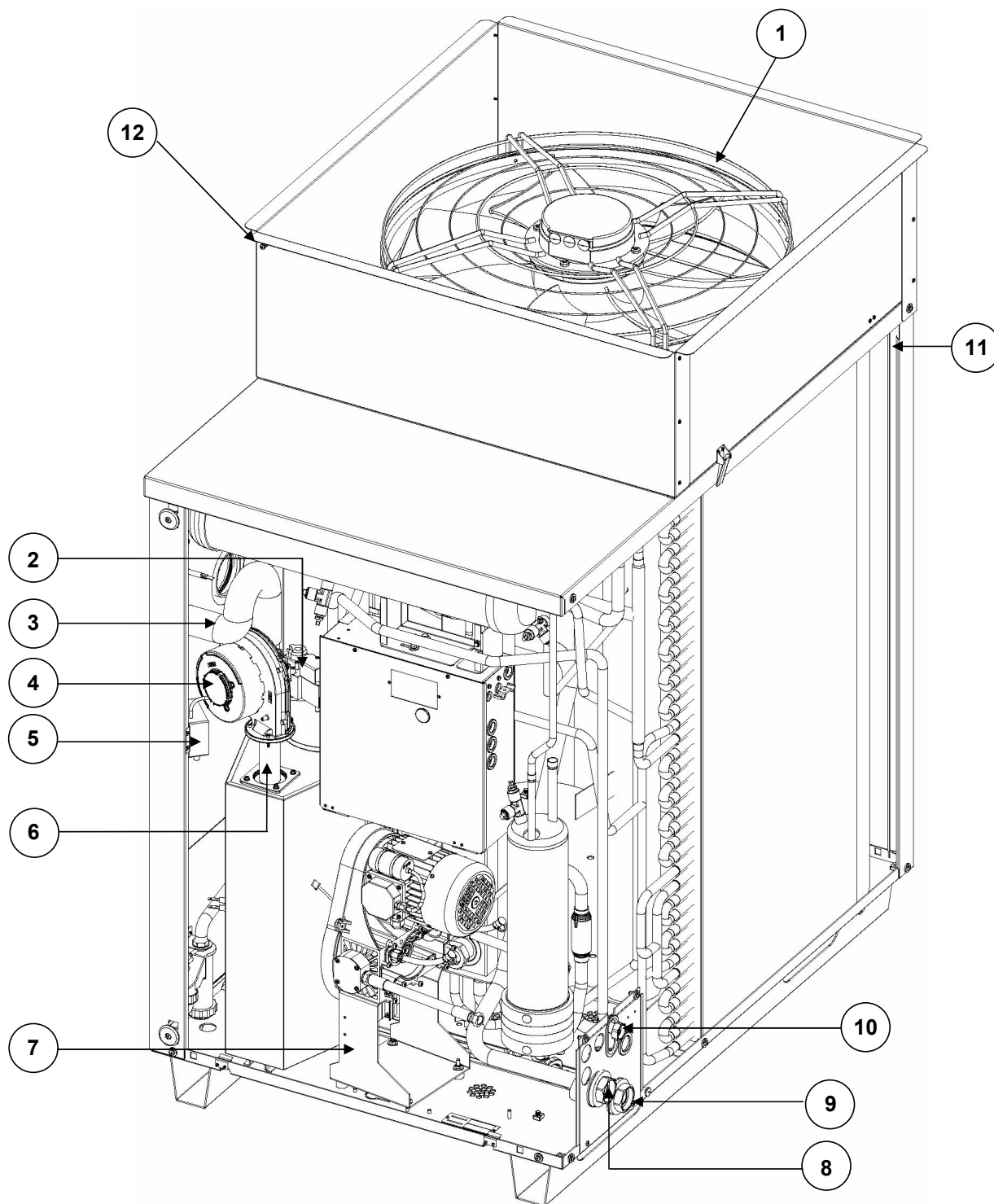
Rysunek 1.3 Elementy wewnętrzne - widok z przodu
