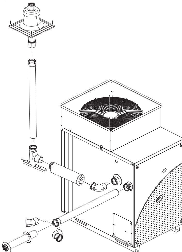
Rysunek 3.3 Odprowadzenie spalin Typu C53 dachowe
